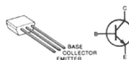
2SC2458 GR Q2, Q3, Q4, Q6
