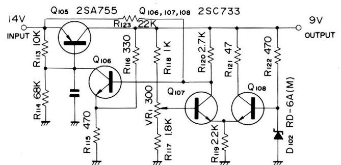
9V AVR
