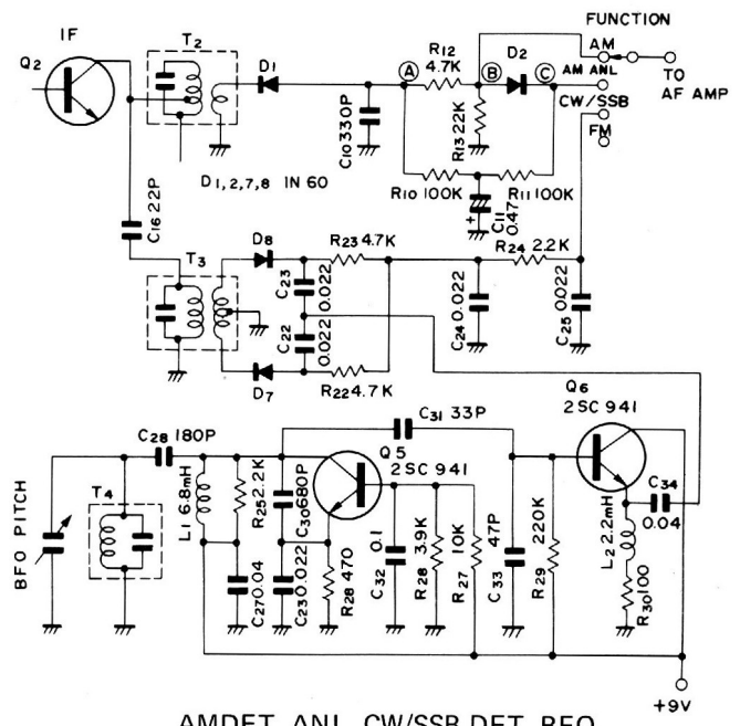
AMDET. ANL. CW/SSB DET. BFO
