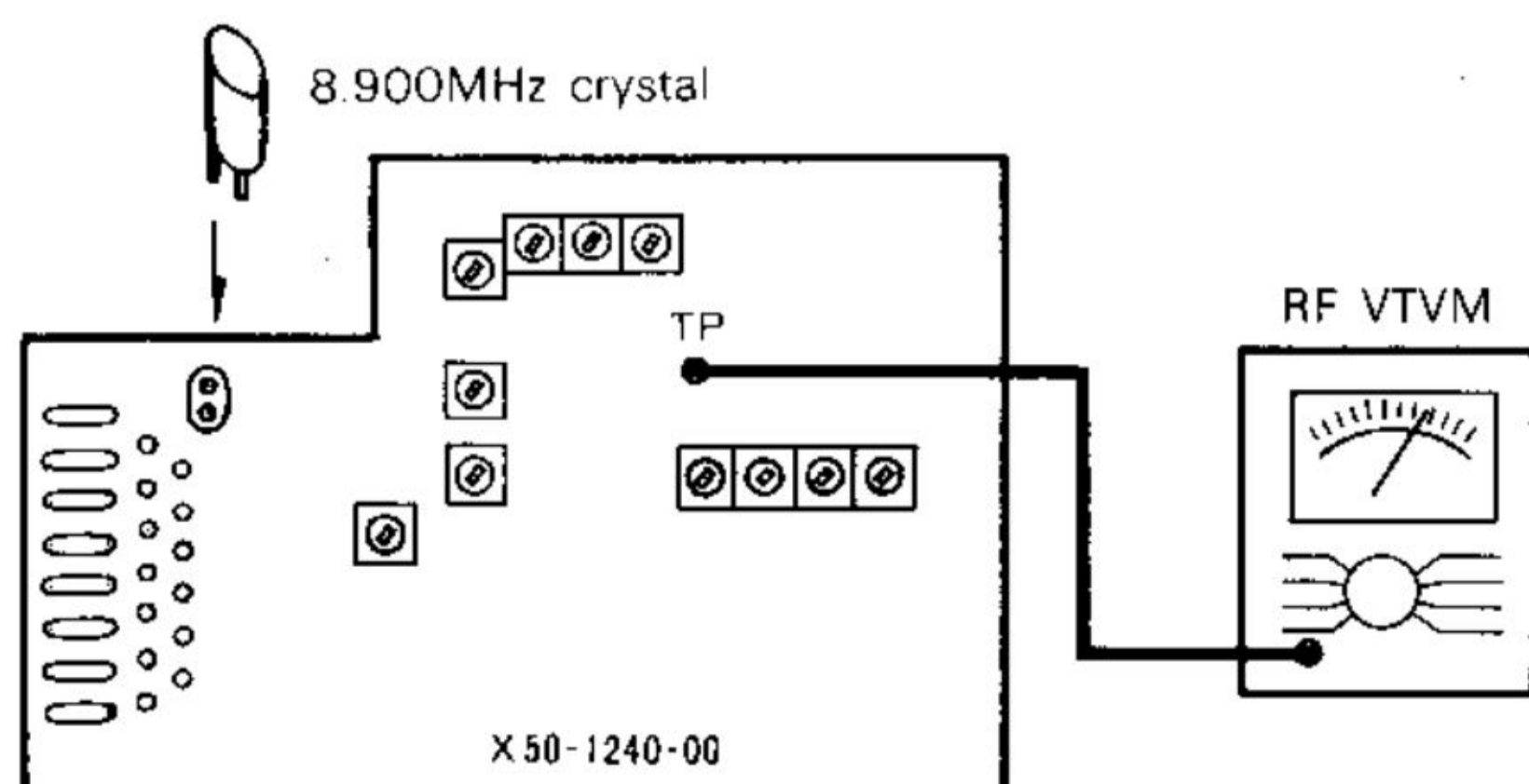
FIG. 6 HET ADJUSTMENT
