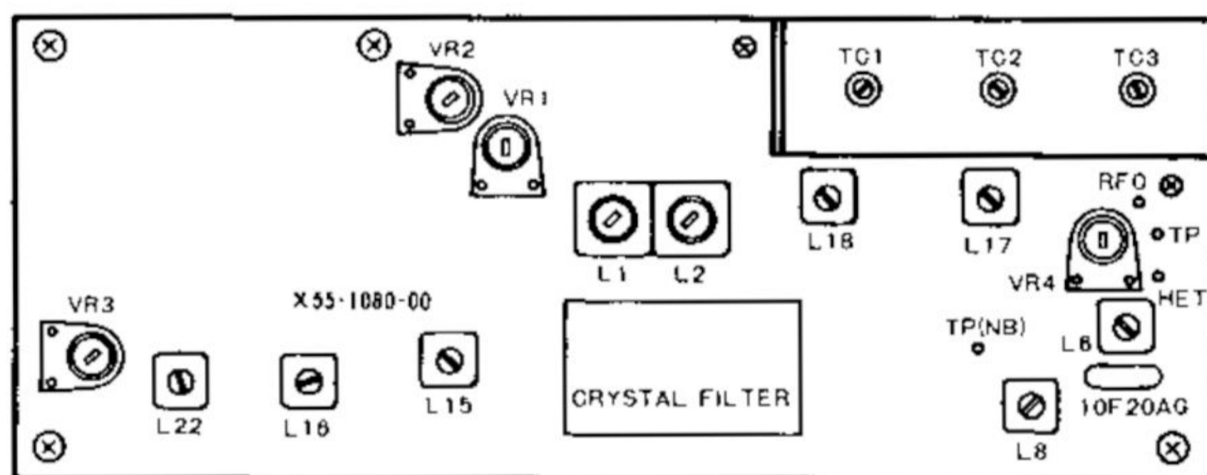
FIG. 15 RX UNIT
