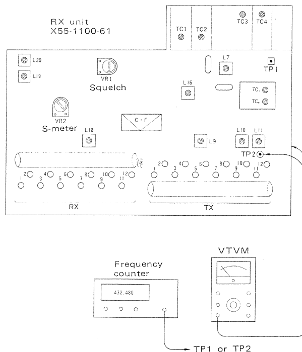
Fig. 6 RX Unit
